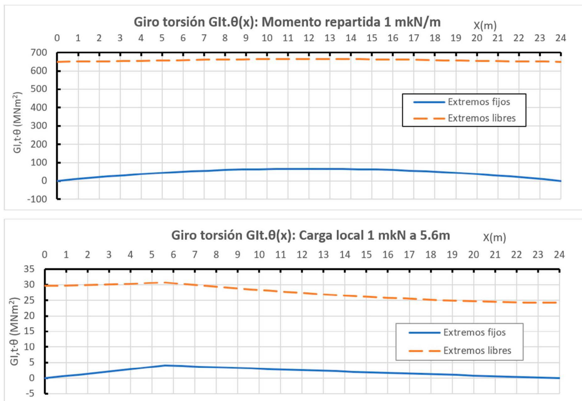
Figura 23. Giros de eje viga para momento repartido y local a ¼ luz.
