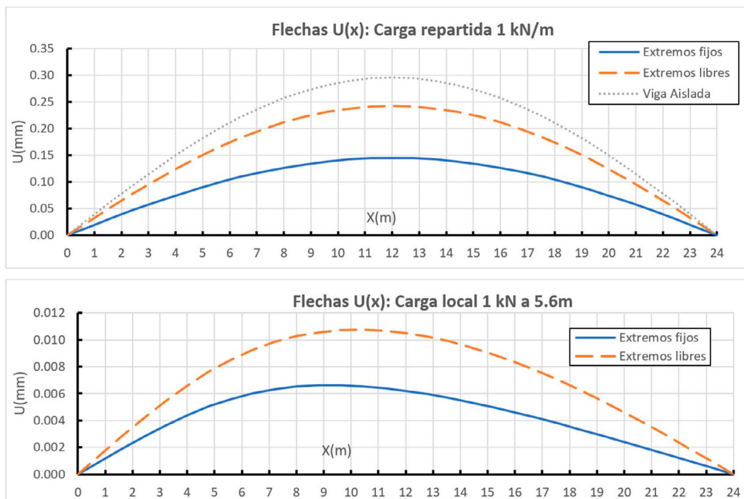
Figura 13: Diagrama de flechas para carga repartida y local a \frac{1}{4} luz.
