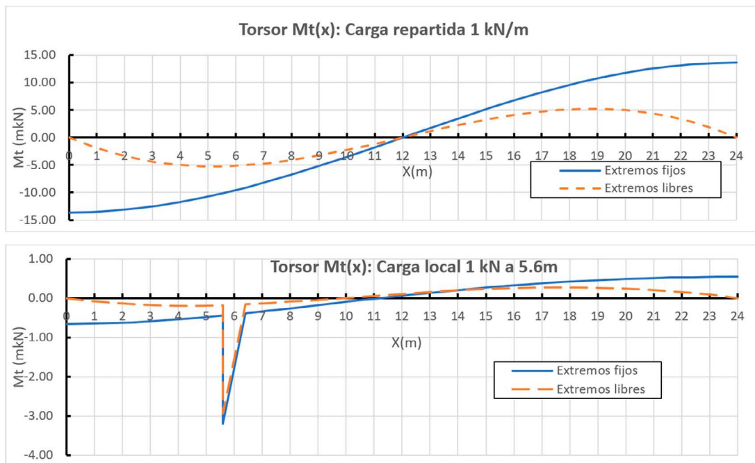
Figura 12. Torsores para carga repartida y local a \frac{1}{4} luz.
