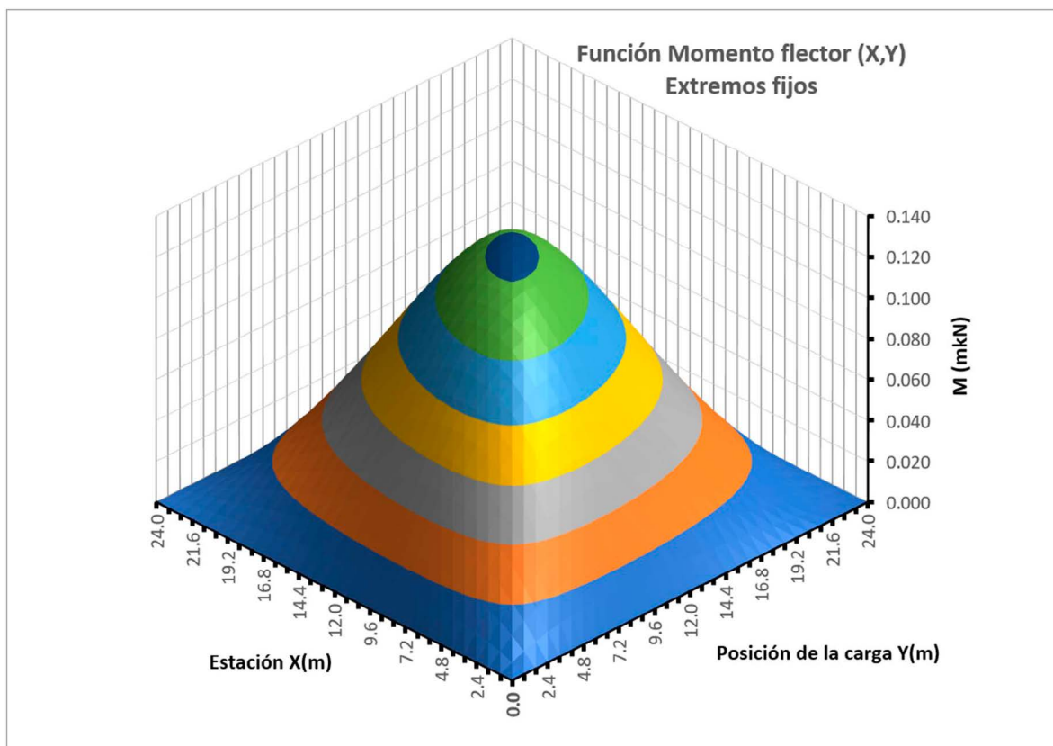
Figura 16. Función de Green de la función de descarga para momento antimétrico y apoyos fijos.
