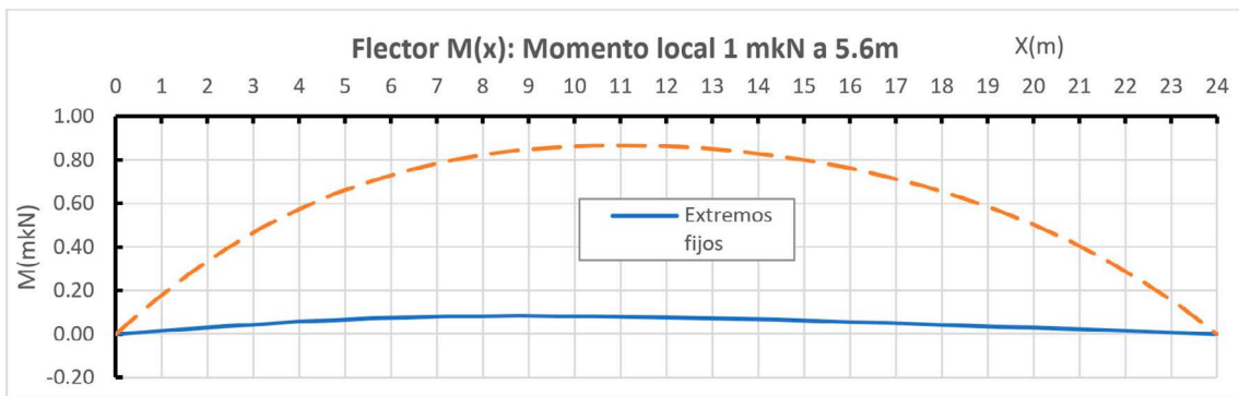
Figura 19. Flectores para momento local a ¼ luz.
