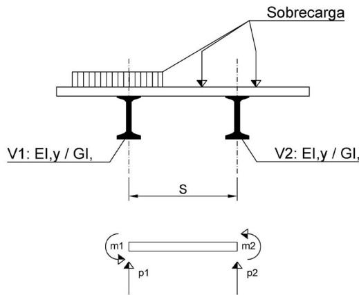
Figura 3. Obtención de reacciones unitarias en el alma de vigas doble T.
