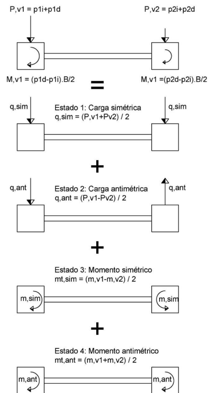
Figura 4. Descomposición de reacciones en unitarias en cuatro estados simples.
