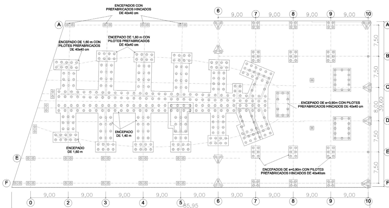
Figura 16. Planta de la cimentación de los edificios Torre y Atrio con pilotes prefabricados hincados.
