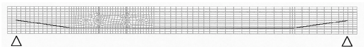
Figura 4. Mallado de la viga V1 incluyendo los elementos tipo cable (en negro).
