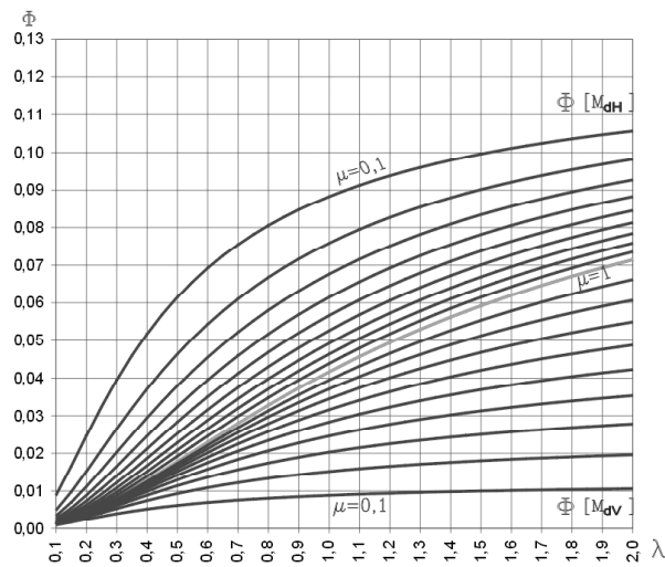
Figura 3. Valores de Φ según EC6 para momentos expresados únicamente en función de L.
