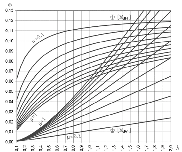
Figura 4. Valores de Φ según DNA para momentos expresados únicamente en función de L.
