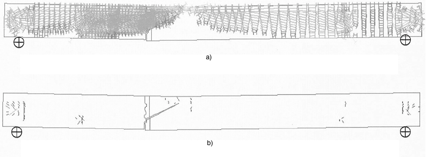
Figura 12. Campos de tensiones principales de compresión; ( |\sigma_{II}| > 2,5 \text{ MPa} ) (a) y de tracción; ( |\sigma_{II}| > 2,5 \text{ MPa} ) (b) obtenidos en el ensayo V1-SFRC-70-FEM-B, bajo carga máxima.
