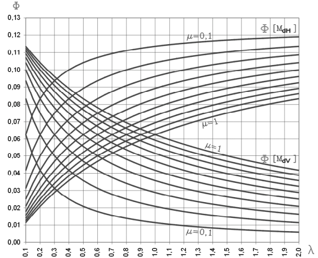
Figura 2. Valores de Φ según DNA para momentos expresados en función de H y L.
