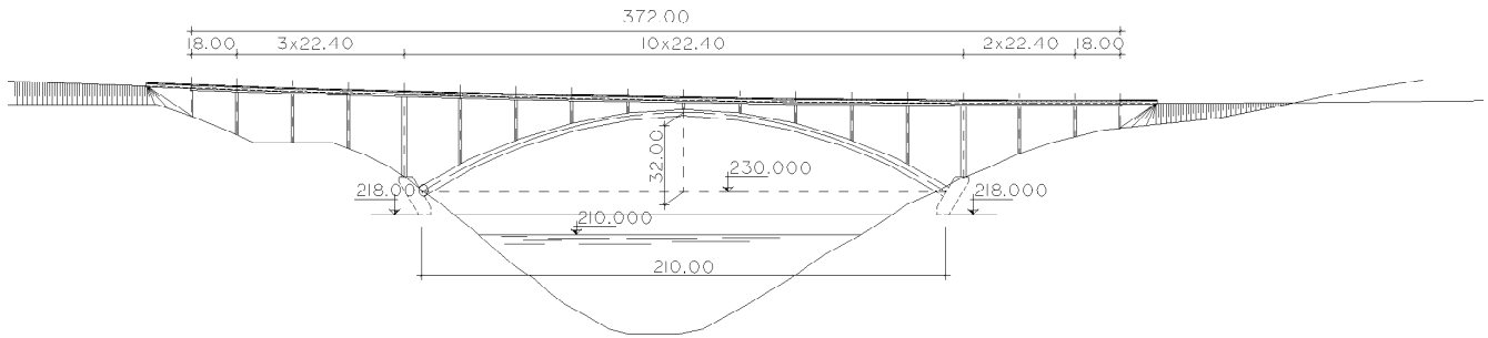
Fig.6. Arco tablero superior. Solución A: Variante de arco en cajón de hormigón armado con luz máxima. Fig.6. Deck arch bridge. Solution A: Variant of a reinforced concrete box arch with maximum span.
