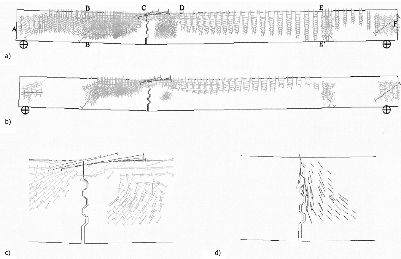
Figura 8. Campo de tensiones obtenido en el ensayo V1-35-FEM bajo carga máxima.
