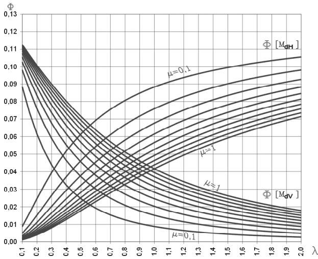
Figura 1. Valores de Φ según EC6 para momentos expresados en función de H y L.
