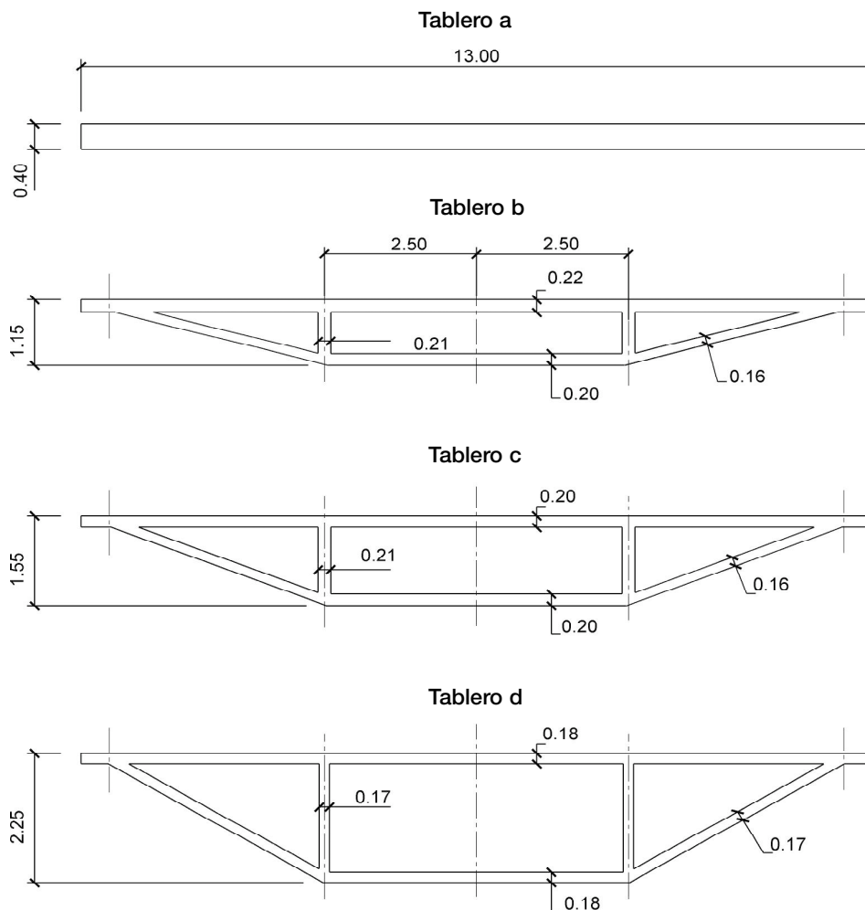
Figura 1. Dimensiones de los tableros.
