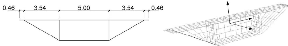
Figura 2. Esquema y mallado de una porción de 1,55m. de longitud de un Modelo Patrón.
