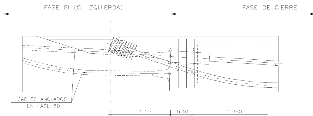
DETALLE DE CRUCE DEL PRETENSADO
