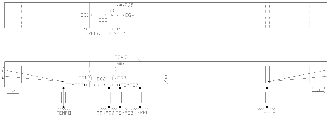
Figura 9. Instrumentación V1-PC.
