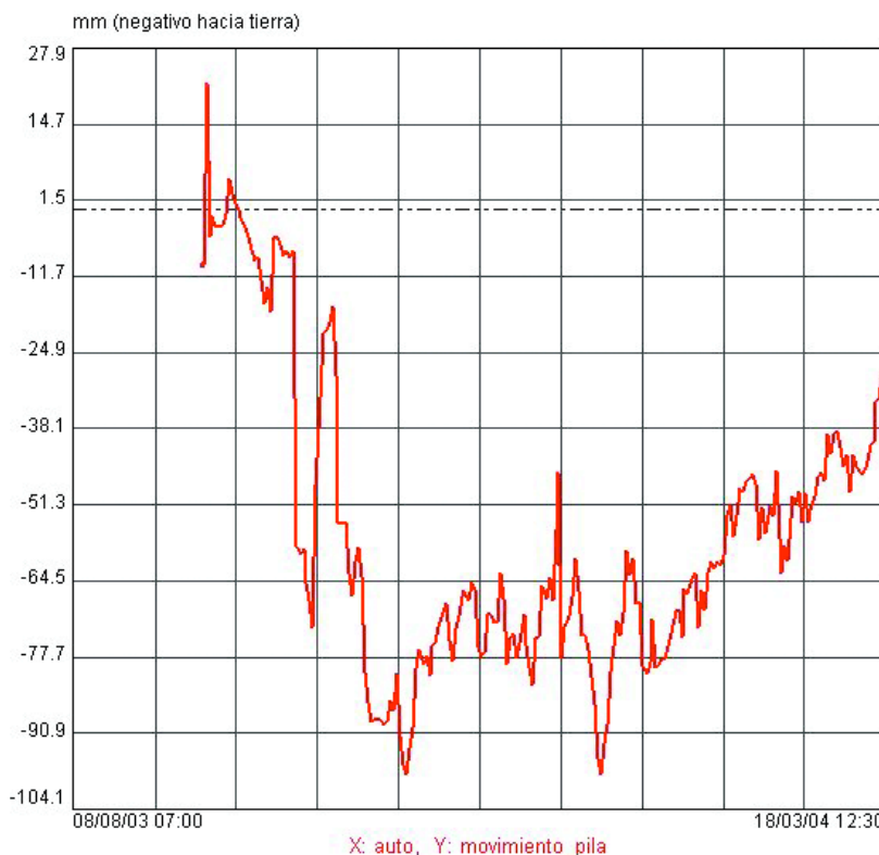
Fig.37. Ejemplo de gráfico acumulado en tiempo real de uno de los sensores controlados. Fig.37. Example of a real time accumulated graph of one of the monitored sensors.
