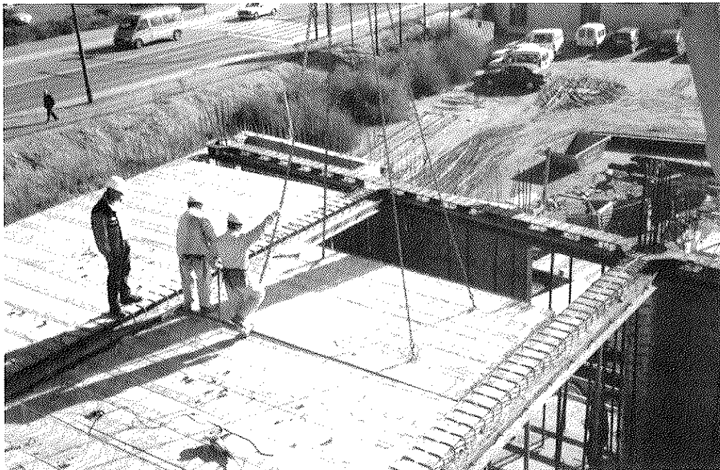
Fotografía 4. Montaje de prelosas apoyadas en jácenas mixtas. Luces 12 x 12 m.
