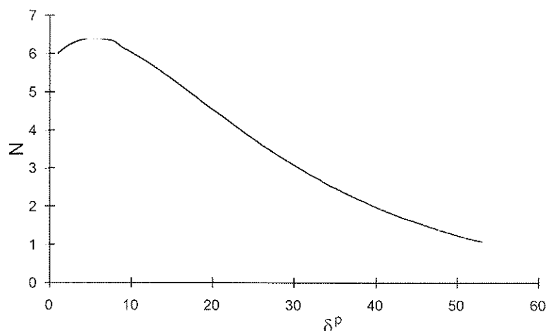
Figura 1. Potencial plástico para el elemento diagonal equivalente.
