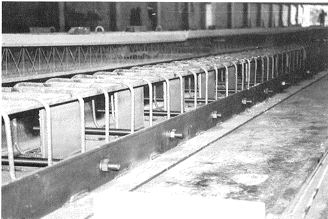
Fotografía 1. Esqueleto metálico.
