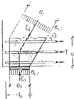
Figura 13: Nudo con varios planos de tirantes
