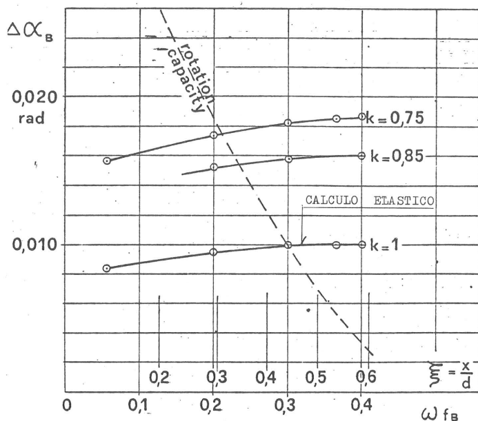
Fig. 15. Comparación entre la rotación plástica necesaria y la capacidad de rotación. MACCHI (3)
