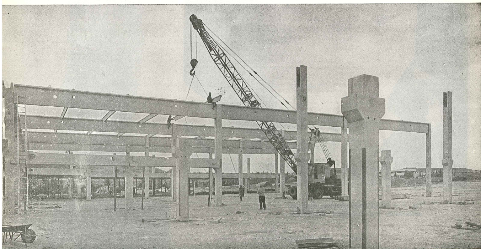
NAVE PREFABRICADA POR CADE
