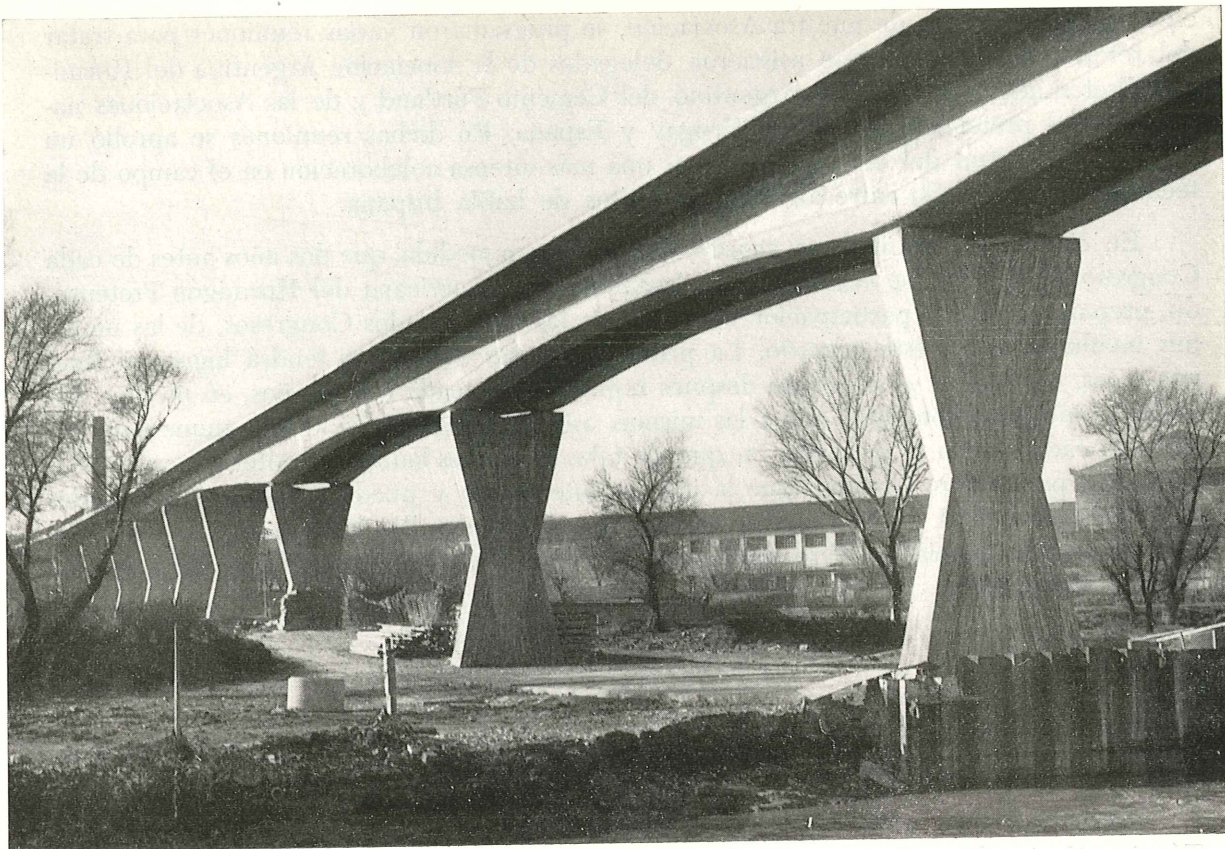
Viaducto Villaverde-Vicálvaro.
