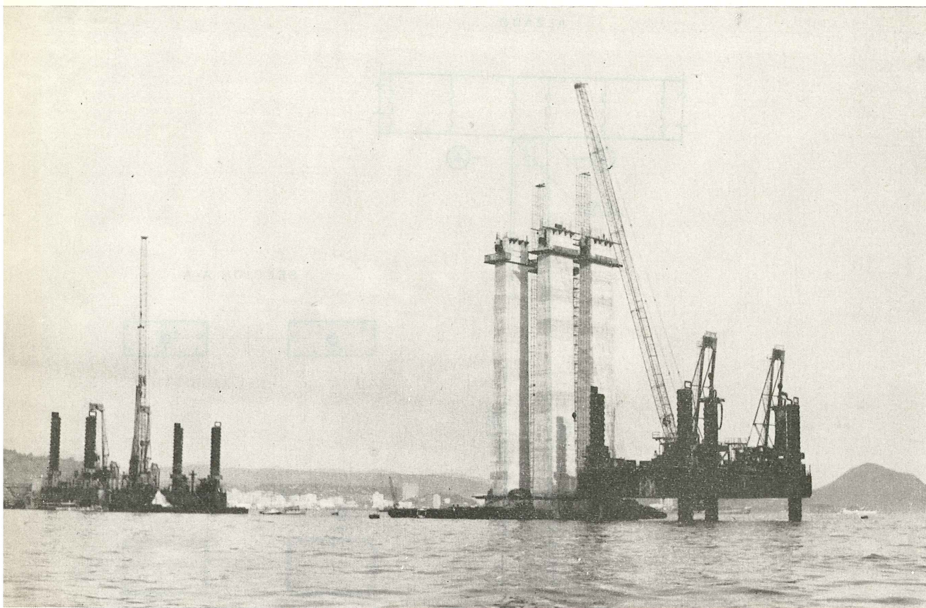
Fig. 19. — Plataformas flotantes y pila P103.
