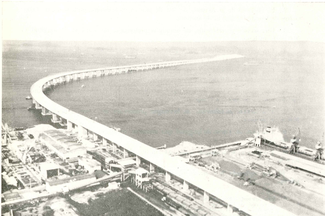
Fig. 2. — Vista del puente desde Río de Janeiro.
