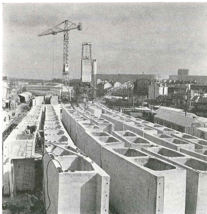
Fig. 65.—Almac n de dovelas.
