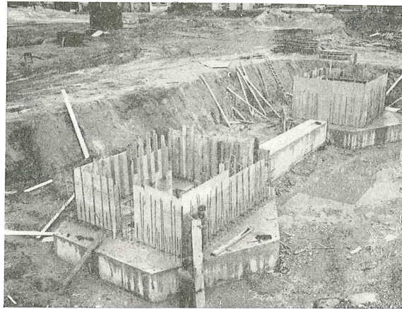
Fig. 47. — Ejecución de los macizos sobre pilotes.
