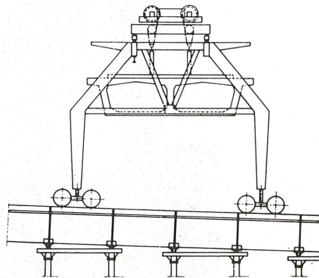
AVANCE DEL PORTICO SOBRE LAS DOVELAS COLOCADAS
