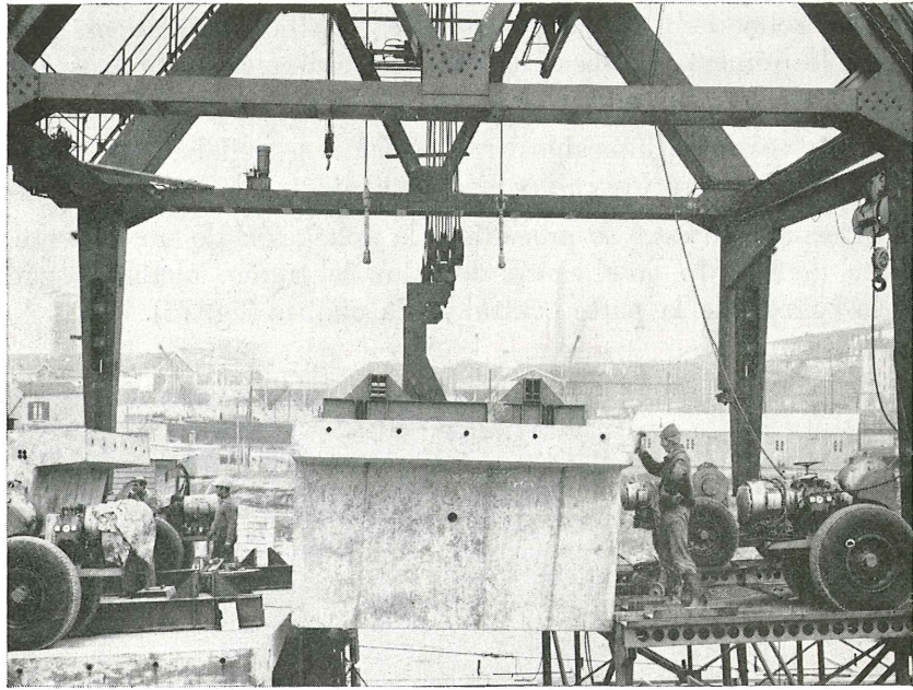
Fig. 71. — Descenso de una dovela.
