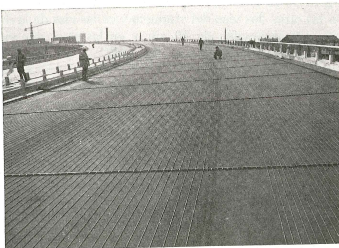
Fig. 108. — Colocación de los cables. Vista general antes de su fijación.
