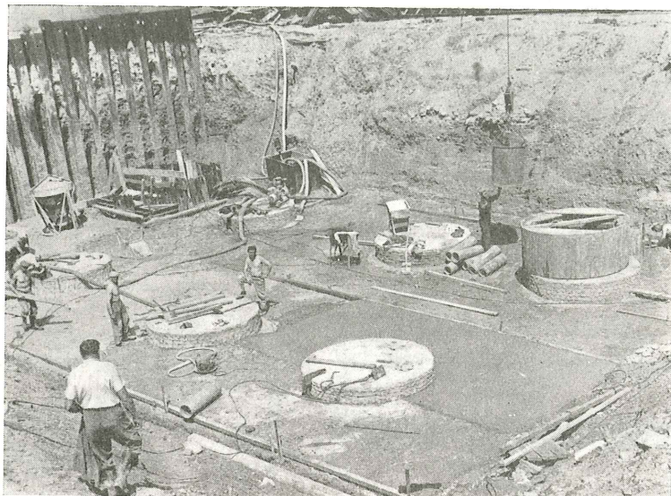
Vista de las cabezas de los pilotes de cimentación para una de las pilas.
