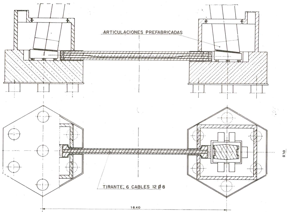
Fig. 48. — Esquema de las zapatas de cimentación.
