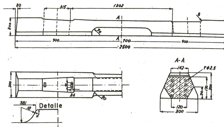
Fig. 1. — Travesía de hormigón pretensado tipo JNBK-75.
