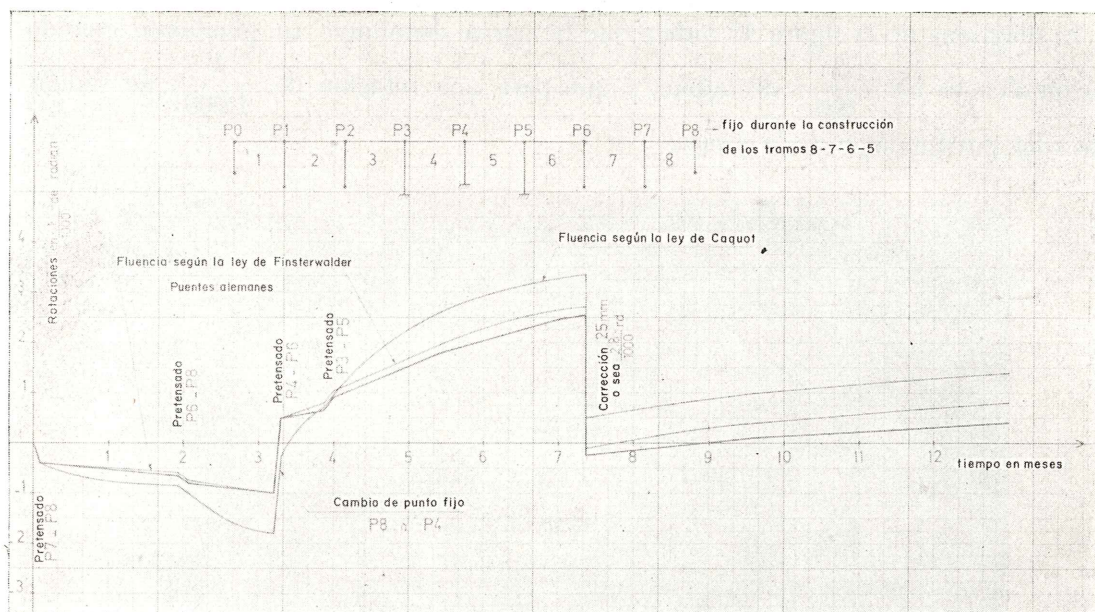
Fig. 46. — Variación de las articulaciones del soporte P7.
