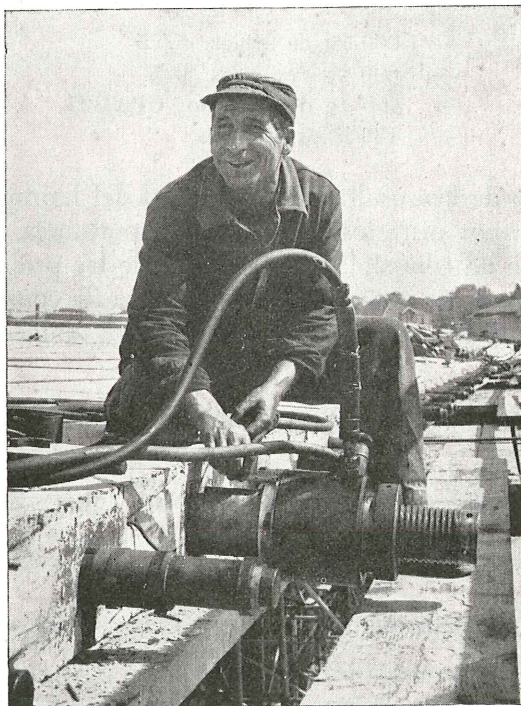
Fig. 79. — Tesado de los cables del forjado superior. En primer plano, anclaje de un cable teso, mantenido en posición mediante las correspondientes cuñas.
