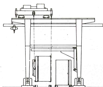
ELEVACION DE LA DOVELA
