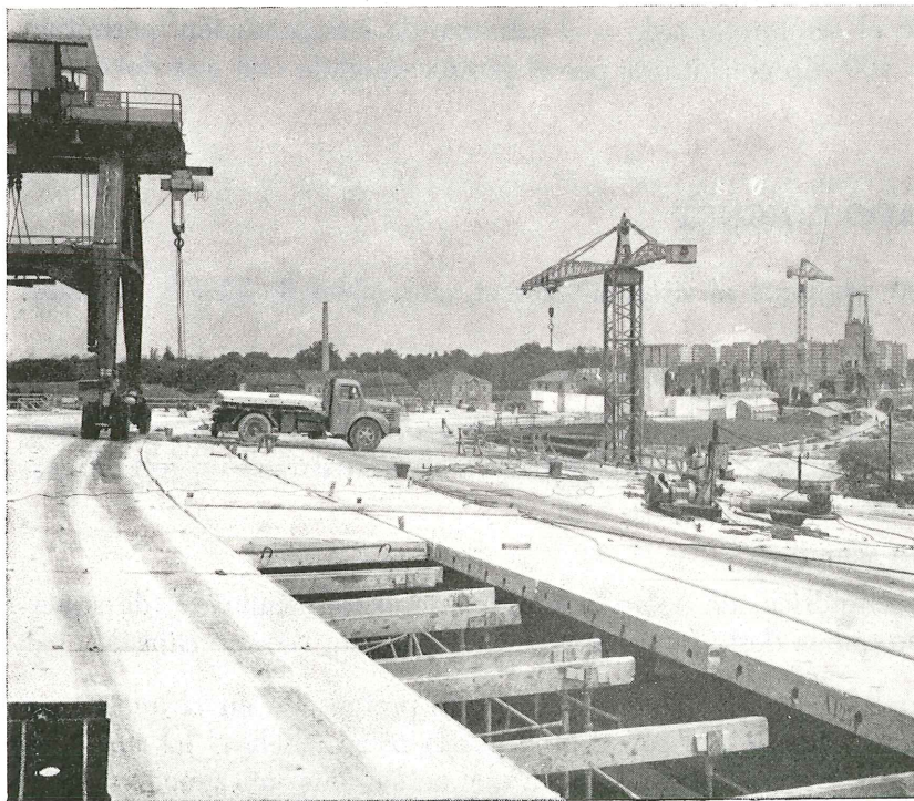
Fig. 72. — Colocación de las placas del forjado.
