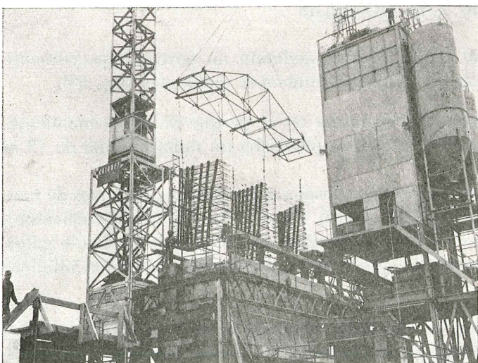
Fig. 61. — Colocación de la armadura de una dovela.
