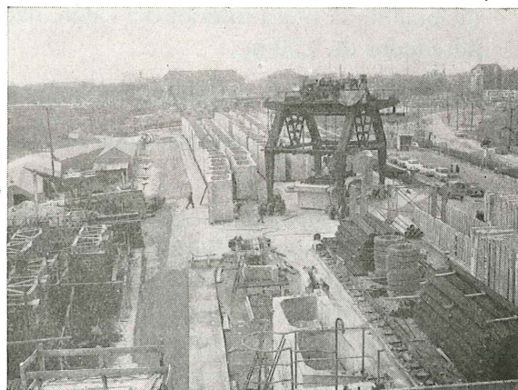
Fig. 24. — Conjunto del parque de almacenamiento en el estribo de Saint-Denis. En primer plano, a la derecha, el almacén de placas de forjado.
