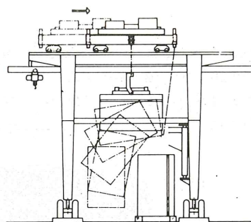
VOLTEO DE LA DOVELA
