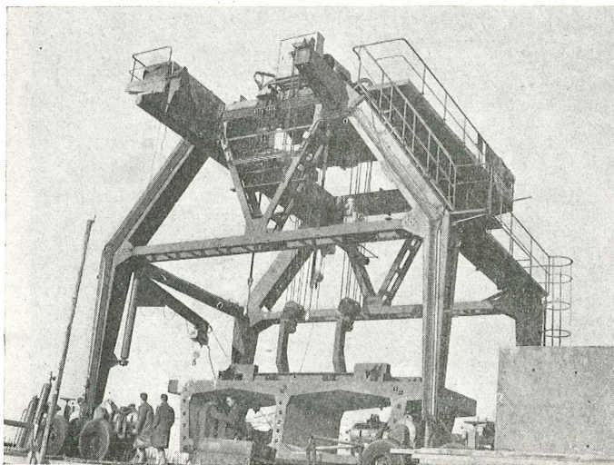
Fig. 67. — Vista de conjunto del pórtico de transporte.
