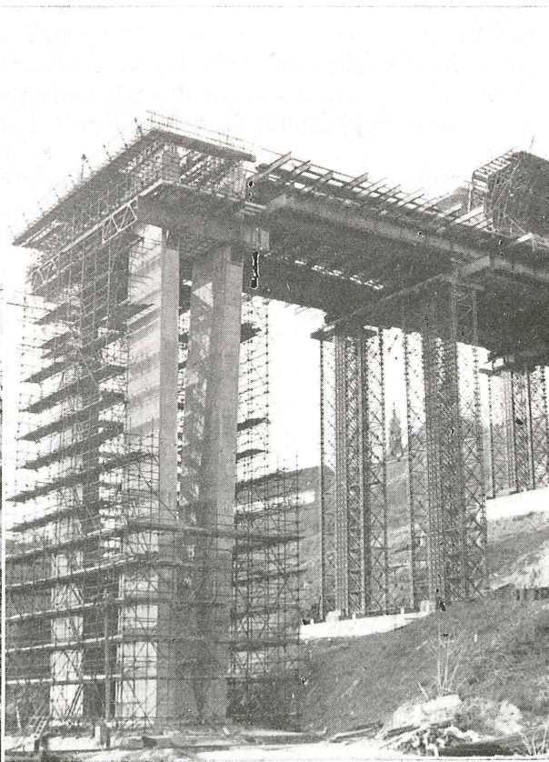
Uno de los tramos extremos, durante su construcción.
