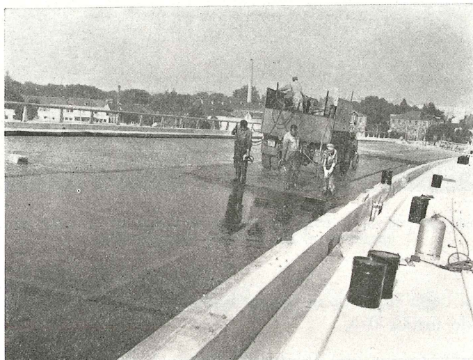
Fig. 104. — Ejecución de la capa de estanquidad, con buen tiempo.
