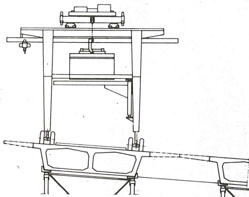
AVANCE DEL PORTICO SOBRE LAS DOVELAS COLOCADAS
