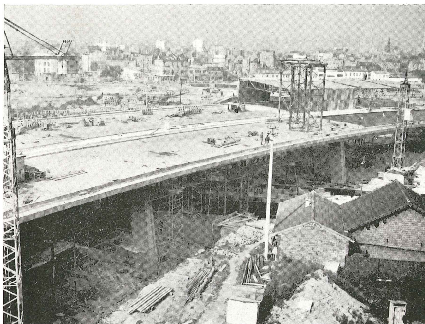
Fig. 105. — Vista general de la obra durante la ejecución de la capa de estanquidad; obsérvese el abrigo móvil de protección.
