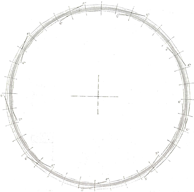
Fig. 12.—Primera capa de aros de pretensado, en el anillo de borde
