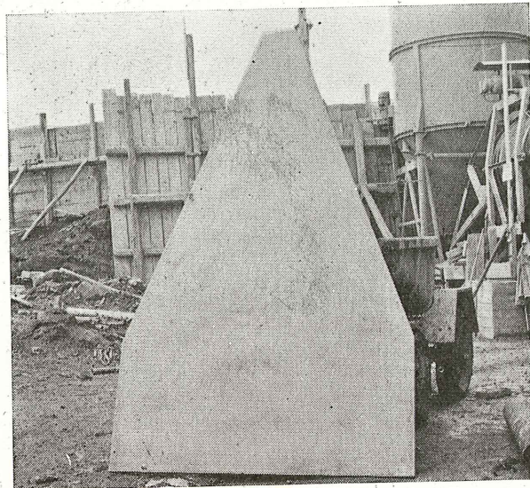
Fig. 19.—Placa de cerramiento, de hormigón armado, prefabricada
