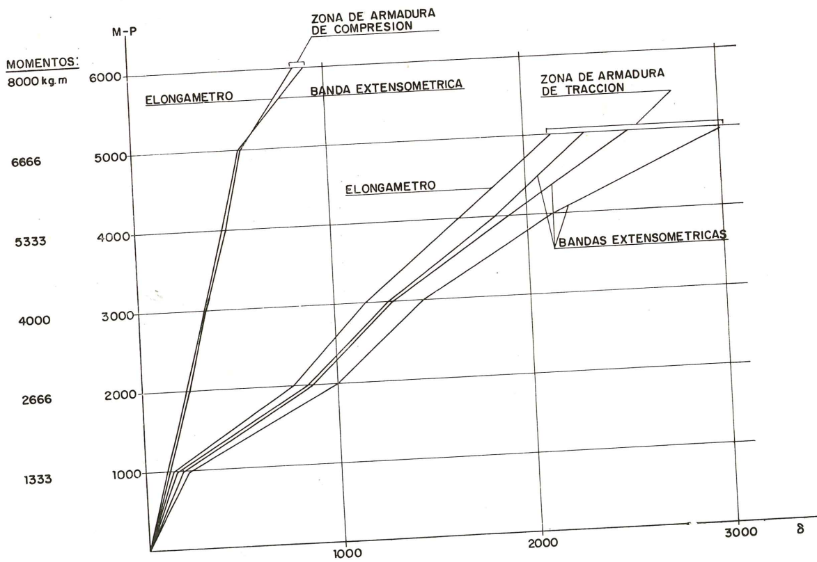
Fig. 38.—Diagramas momento-rotación en secciones central y lateral
