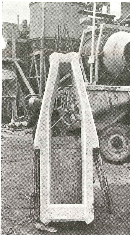
Fig. 15.—El elemento 1, de hormigón armado prefabricado
