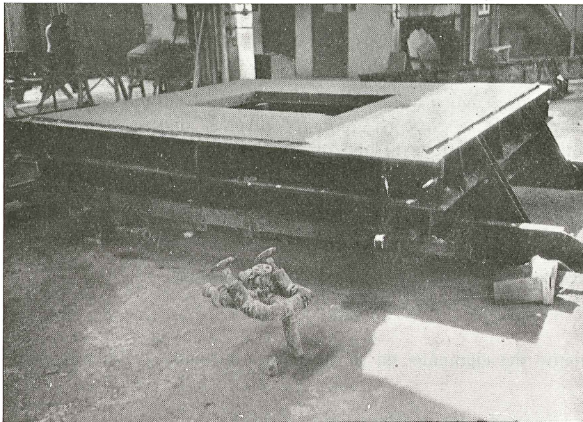
Panel, con hueco de ventana, hormigonado en molde horizontal.
