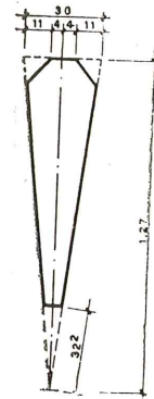
Fig. 9.—Placa prefabricada de cerramiento entre los elementos 1
