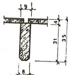
Fig. 8.—Apoyo de la placa sobre el nervio del elemento 1
