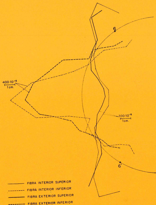
Fig. 26.—Deformaciones zona central (Elongámetro) (fase 3)
