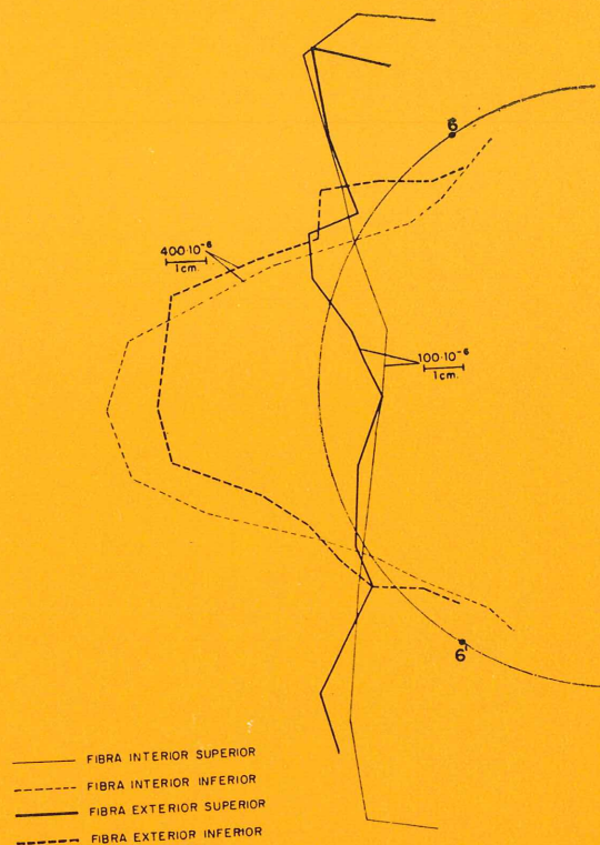
Fig. 27.—Deformaciones zona central (Elongámetro) (fase 4)
