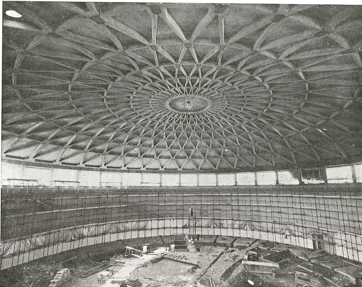
Fig. 25.—Vista, desde el interior, de la cúpula terminada
