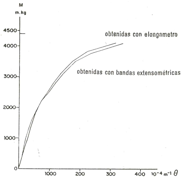
Fig. 30.—Viga testigo número 1. Ley de momentos-rotaciones.
