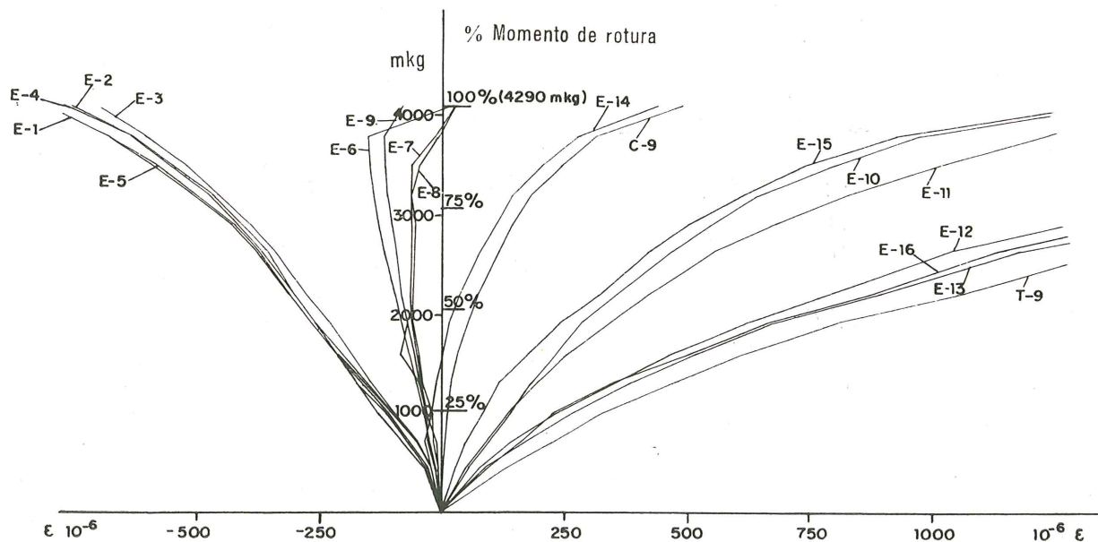
Fig. 28 b).—Deformaciones - Elongámetro.
