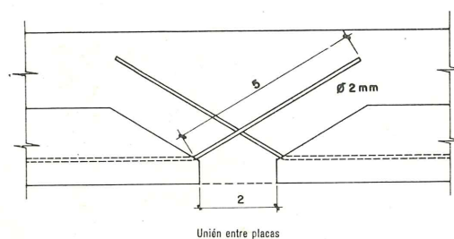
Fig. 4 a)-1.—Sección a-a. Cotas en centímetros.
