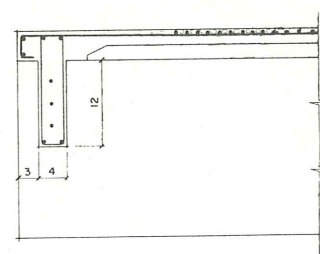
Fig. 4 a)-1.—Sección a-a. Cotas en centímetros.
