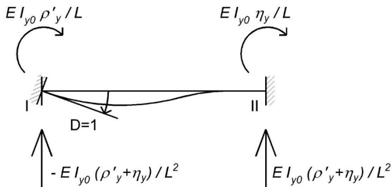
Figura 5. Coeficientes de rigidez por giro unitario en un extremo.
