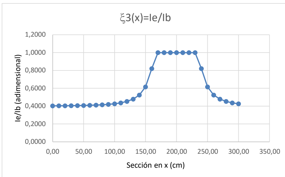
Figura 14. Gráfica de rigideces relativas en soportes 1-3 y 2-4.
