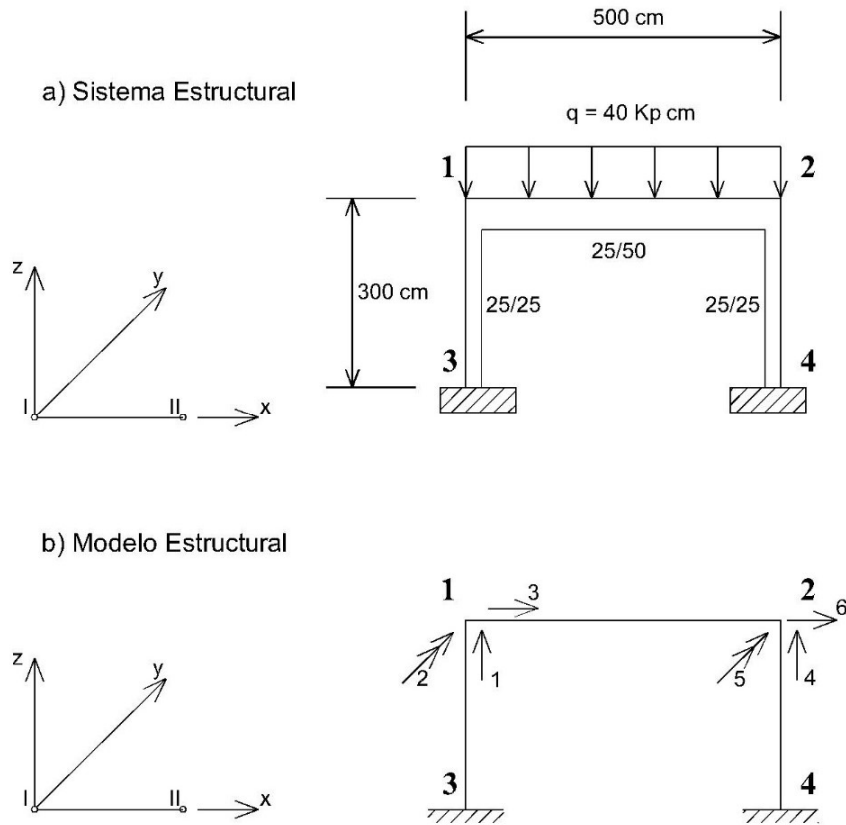
Figura 11. Pórtico y Modelo Estructural.
