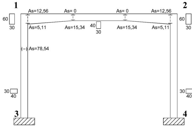
Figura 10. Secciones de armaduras necesarias.
