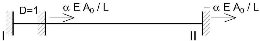
Figura 2. Coeficientes de rigidez por desplazamiento longitudinal unitario en un extremo.
