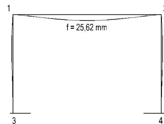
a) Gráfica de Movimientos
