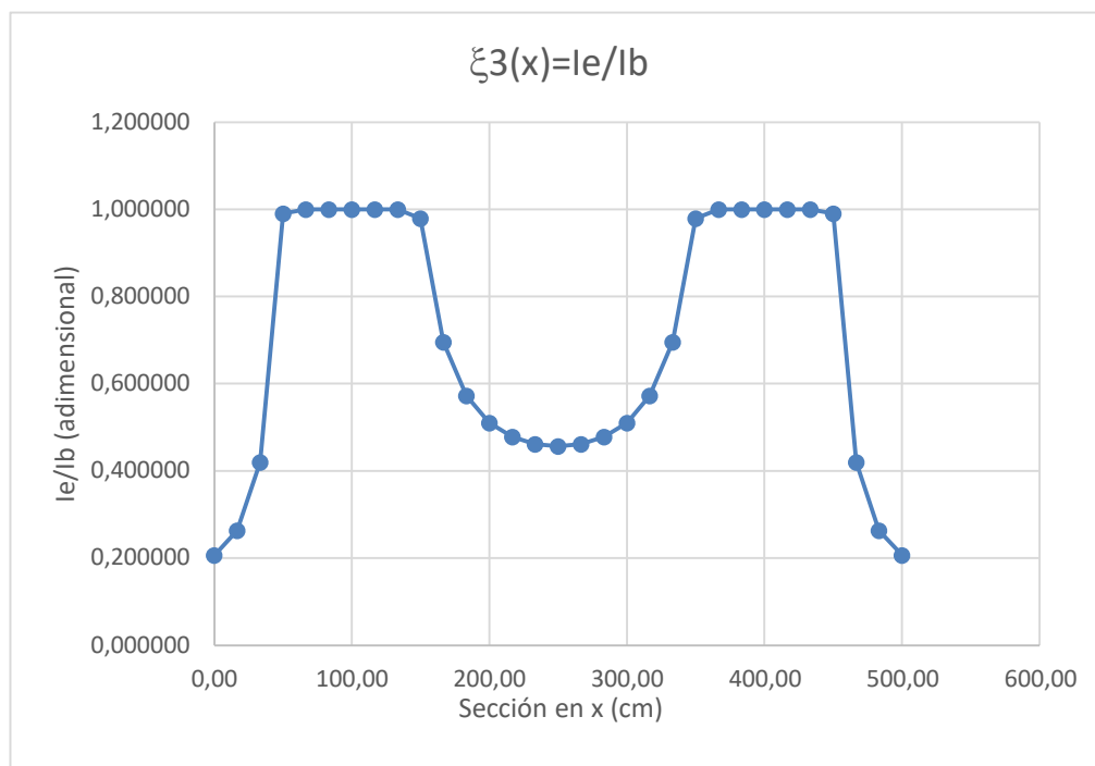
Figura 13. Gráfica de rigideces relativas.
