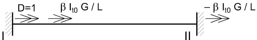
Figura 3. Coeficientes de rigidez por giro longitudinal unitario en un extremo.
