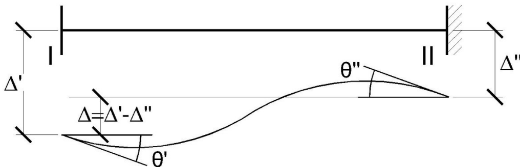
Figura 4. Barra con giros y traslaciones de extremo.
