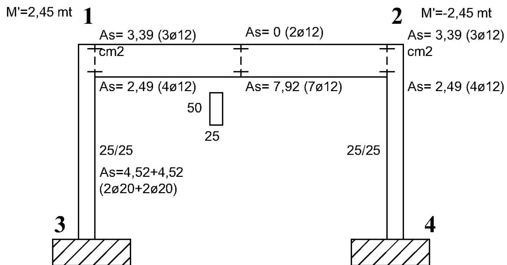
Figura 12. Secciones de armaduras necesarias.
