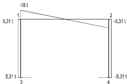
b) Gráfica de esfuerzos Cortantes
