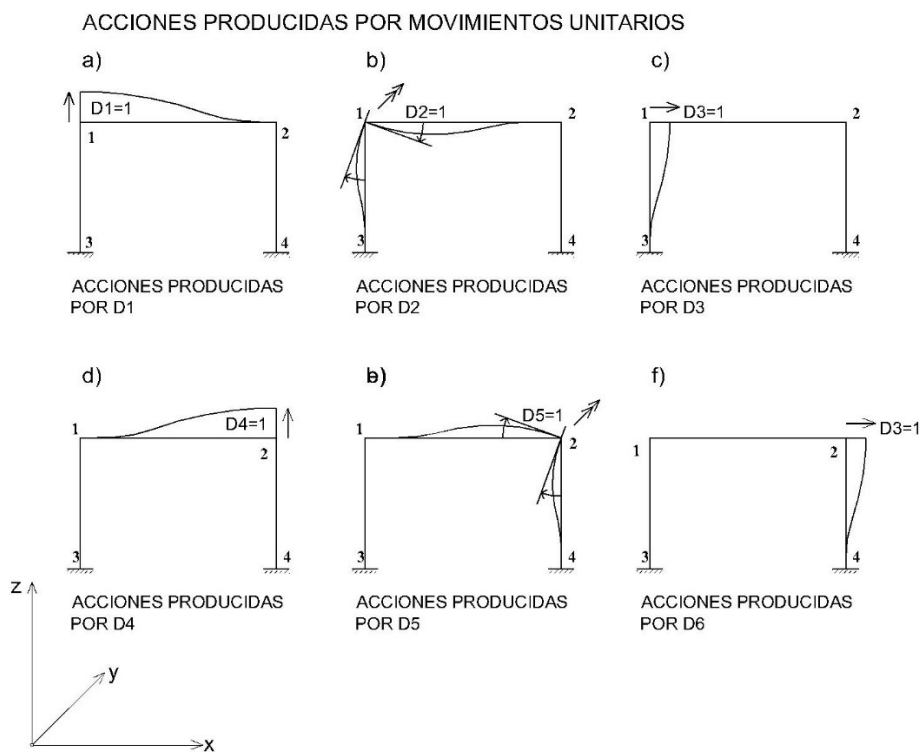
Figura 8. Movimientos unitarios para el cálculo de los coeficientes de rigidez.
