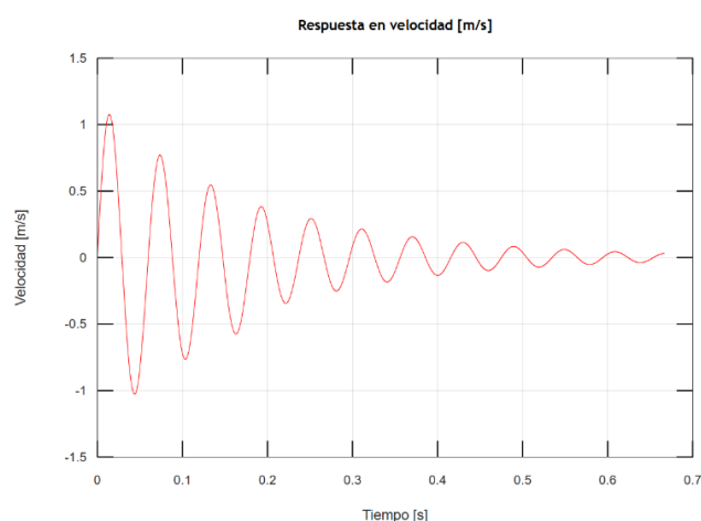
Figura 22. Respuesta en Velocidad del sistema SDOF.
