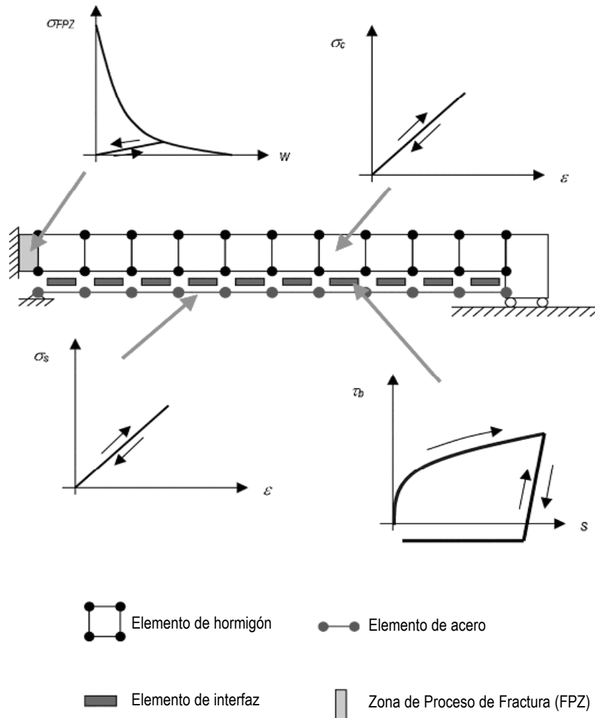
Figura 3. Modelo de elementos finitos del tirante de hormigón armado.
