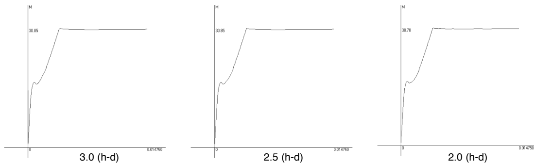
Figura 14. Resultados obtenidos considerando la rigidización por rozamiento en la interfaz para diferentes profundidades de bloque de hormigón traccionado.
