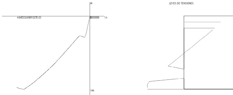
Figura 16. Comportamiento de la sección mixta con chapas capaces de resistir compresión y tracción.
