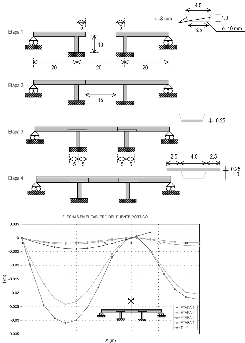
Figura 21. Estructura hiperestática.
