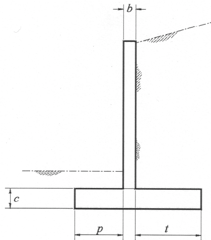
Figura 3. Representación de las variables geométricas.
