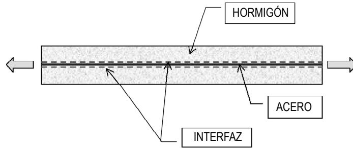
Figura 1. Tirante de hormigón armado.
