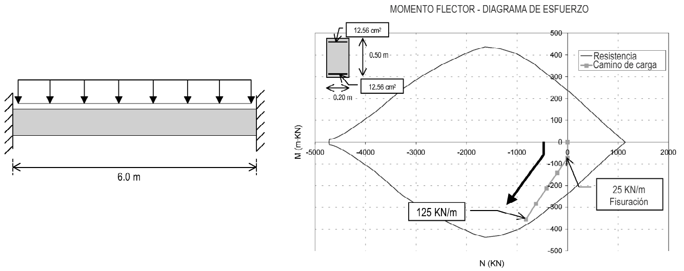
Figura 20. Fenómeno de acoplamiento elongación – curvatura.
