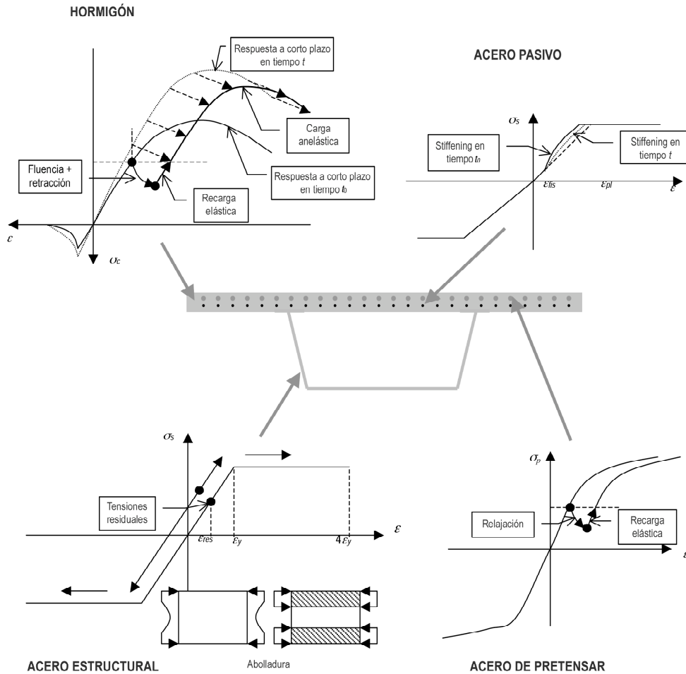
Figura 7. Modelos de comportamiento de los diferentes materiales.
