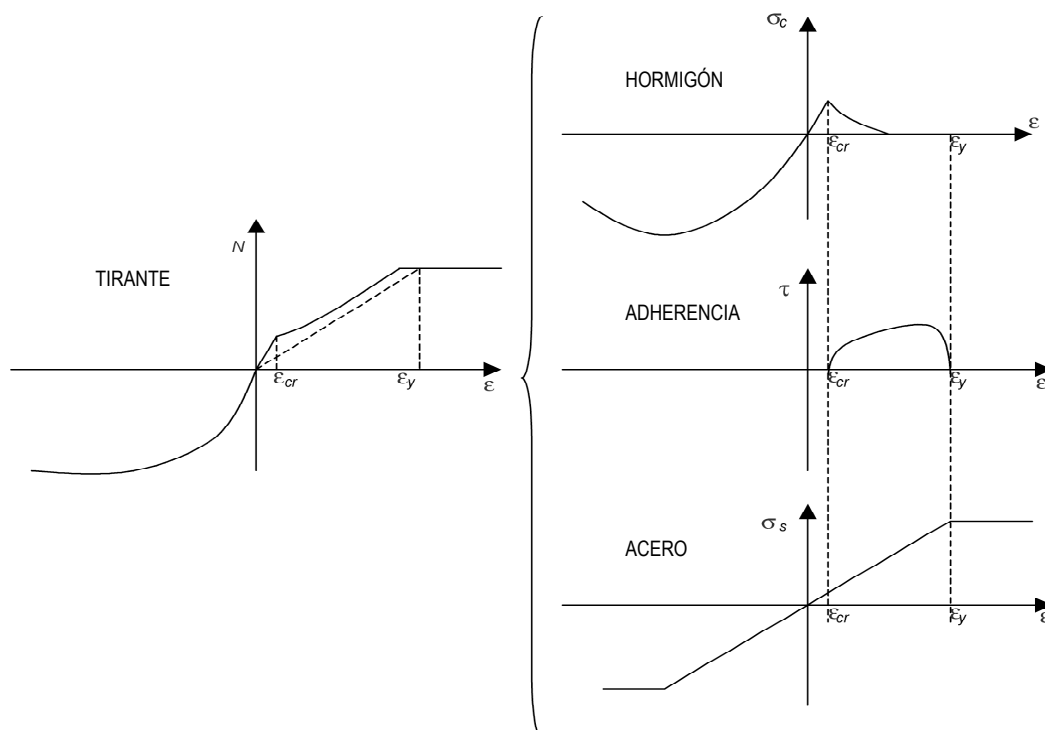
Figura 2. Comportamiento en compresión y tracción del tirante.
