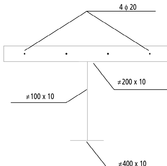
Figura 15. Sección mixta.
