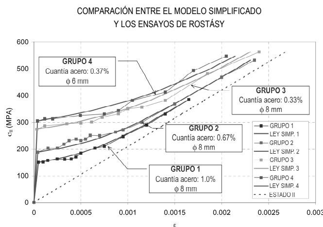
Figura 6. Comparación con los resultados experimentales de Rostásy.
