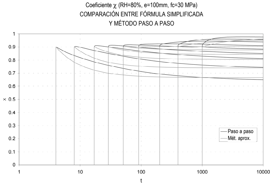
Figura 9. Fórmula aproximada para el cálculo del coeficiente \chi .
