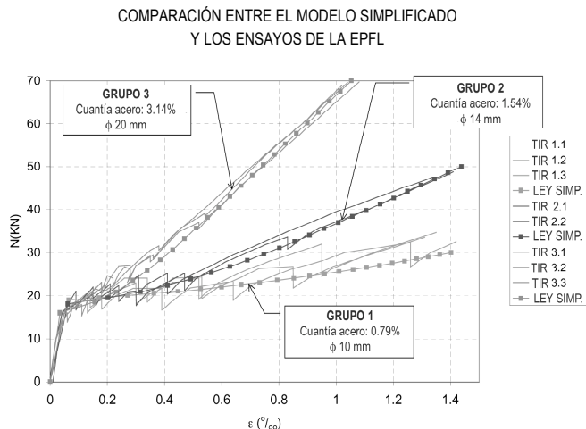
Figura 5. Comparación con los resultados experimentales de la EPFL.
