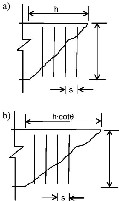
Figura 2. a) Estribos 90° y bielas a 45° b) Estribos a 90° y bielas a θ.
