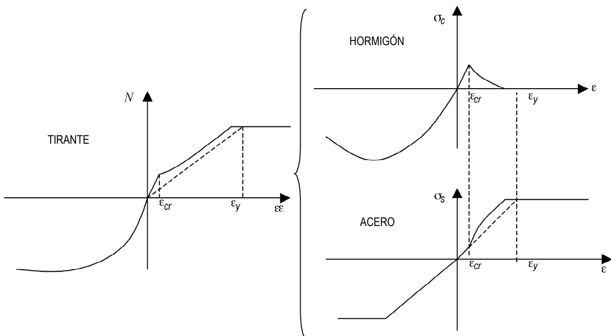
Figura 12. Efecto del tension - stiffening reproducido con acero y hormigón.
