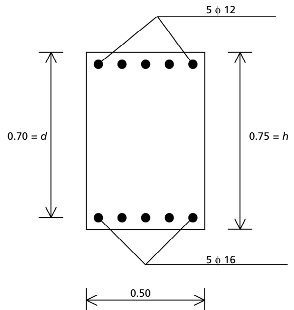
Figura 10. Sección de hormigón armado.
