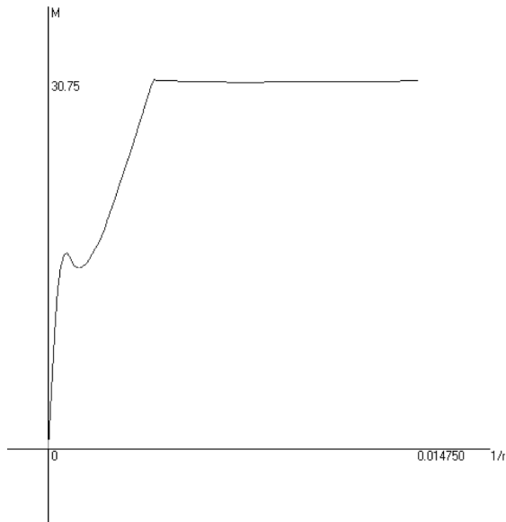
Figura 13. Resultado despreciando la contribución del rozamiento.
