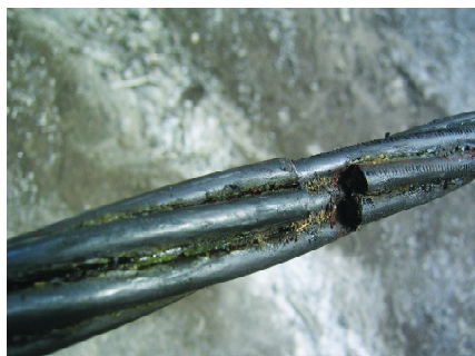
Figura 19. Alambres seccionados. Figure 19. Split wire strands.
