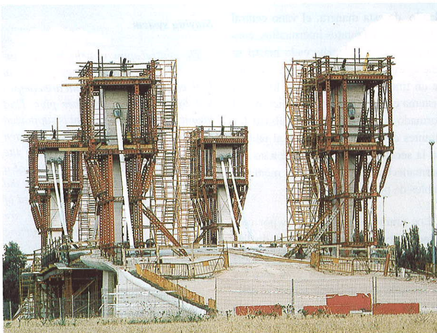
Figura 14. Andamios para el tesado de tirantes. Figure 14. Cables prestressing falseworks.
