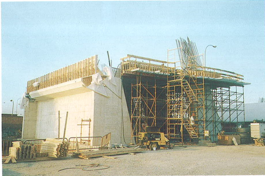
Figura 15. Estribo. Figure 15. Abutment.
