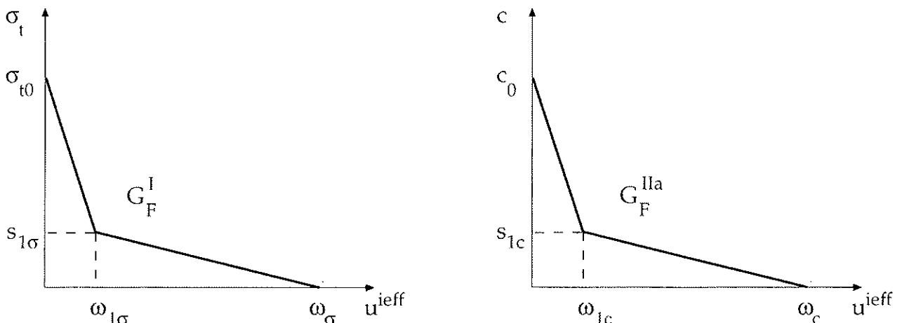
Figura 10. Funciones de ablandamiento bilineal: (a) resistencia de la intercara en la dirección normal al alambre, (b) cohesión entre el alambre y el hormigón.
