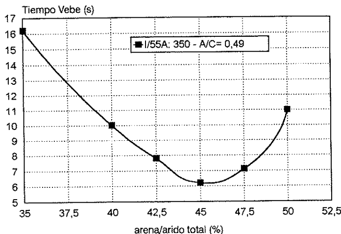
Figura 7. Consistometrías para optimización de esqueleto granular y relación agua/cemento para I/55A.
