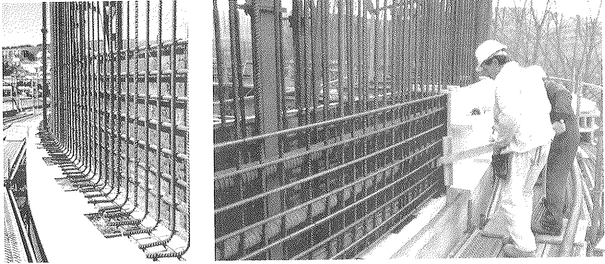
Figura 22. Apoyos de neopreno sobre la estructura de hormigón de base del fuste, armaduras activas y pasivas pertenecientes a la parte inferior del fuste. Inicio del montaje del encofrado deslizable.
