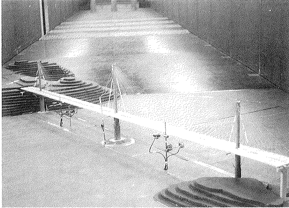
Fig. 13 Ensayo del modelo completo en túnel de viento.
