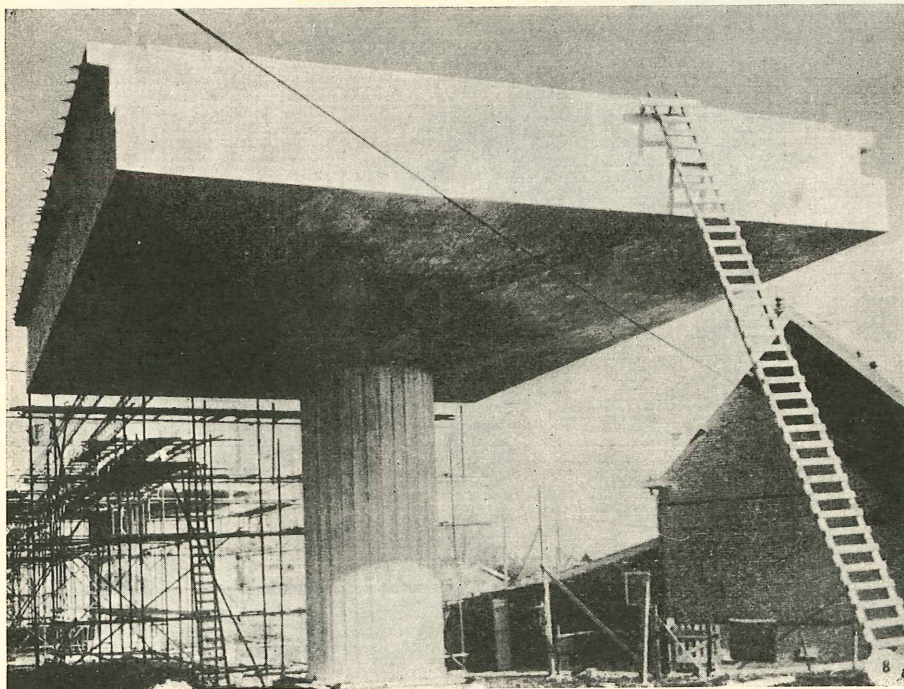
Fig. 8.—PUEBTE BODEGRAVEN, HOLANDA
