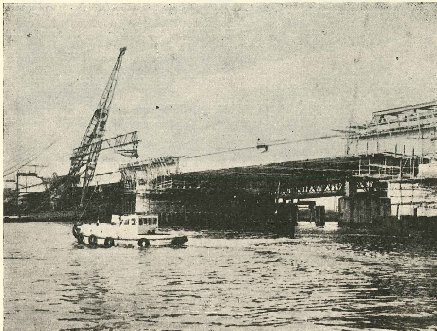
Fig. 7. — PUEBTE EN ROERMOND, HOLANDA
