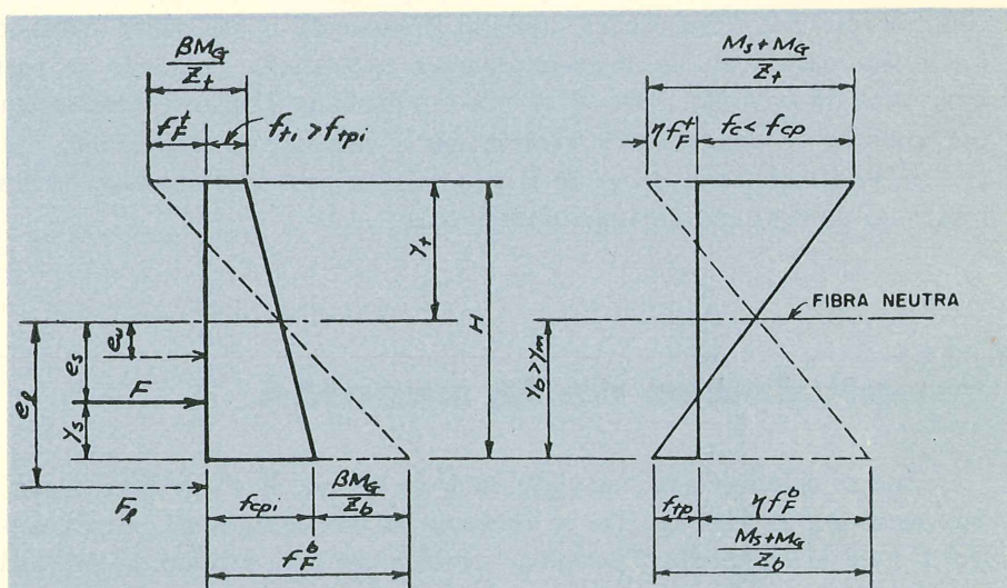
Fig. II.—Distribución de tensiones en el caso en que se verifique Z_b = Z_m , y_b > y_m y e_u < e_s < e_l .
