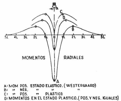
MOMENTOS MAXIMOS EN EL PAVIMENTO ESTADOS ELASTICOS Y PLASTICOS
