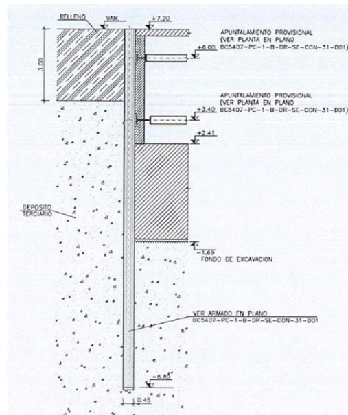
Figura 16. Esquema en alzado de los principales elementos de apuntalamiento para la Torre B.
