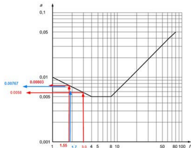
Figura 9. Aceleración límite de referencia según la frecuencia, a multiplicar por un factor 200 o 400.
