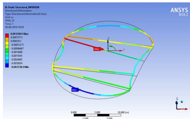
Figura 18. Deformación escalada del sistema de apuntalamiento.
