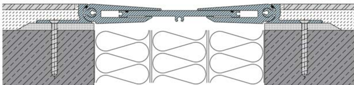
Figura 24. Esquema de junta utilizada en forjados de hormigón entre nuevas torres y estadio.
