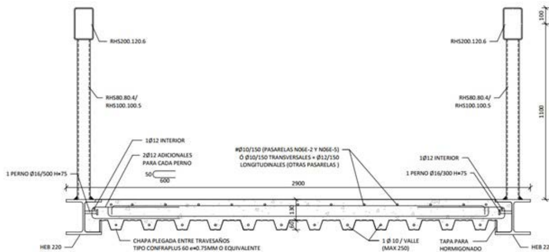
Figura 27. Sección tipo de las pasarelas.
