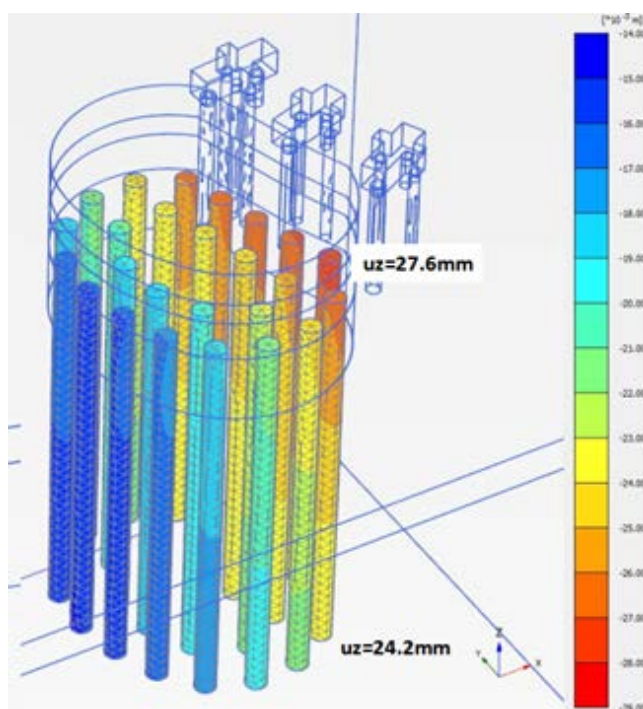
Figura 14. Ejemplo de resultados de movimientos verticales en los pilotes, en una combinación en ELS, en el modelo de PLAXIS.
