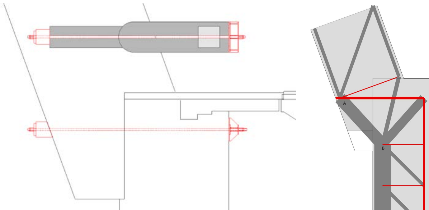
Figura 5. Refuerzo de las costillas. Barra pretensada (i) y esquema de bielas y tirantes. El recrecido del tacón permite bajar el nudo B y mejorar además la dimensión de la biela AB.
