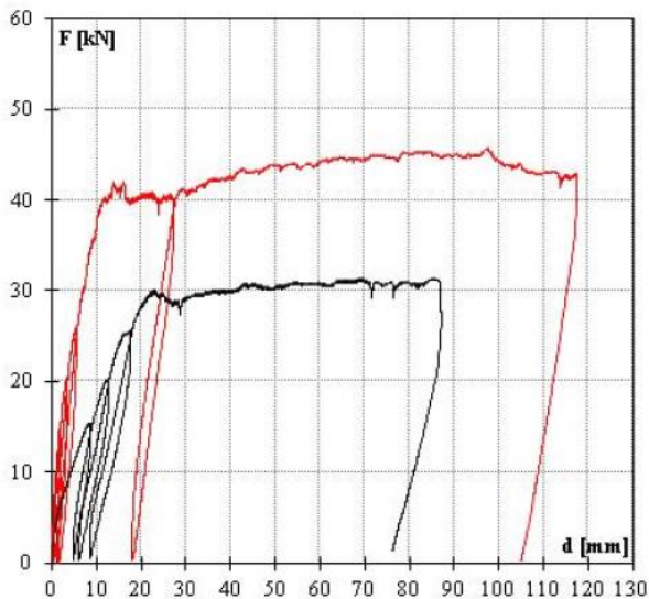
Figura 9. Curvas Carga-flecha central
