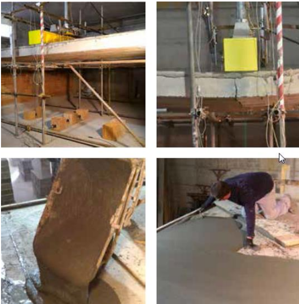
Figura 8. Ensayo sobre forjados
