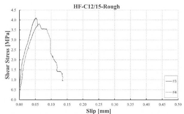
Figura 5. Diagrama tensión rasante - desplazamiento
