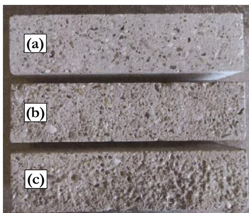
Figura 3. Rugosidad de las probetas de hormigón
