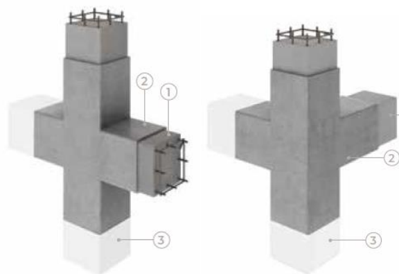
Figura 13. Esquema de refuerzo de nudos
