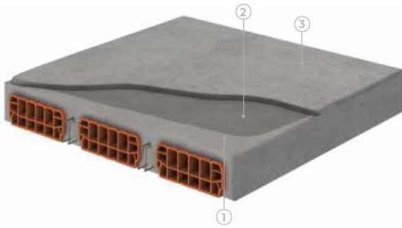
Figura 14. Esquema de refuerzo de forjados
