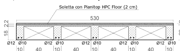
Figura 7. Sección del forjado con capa de refuerzo
