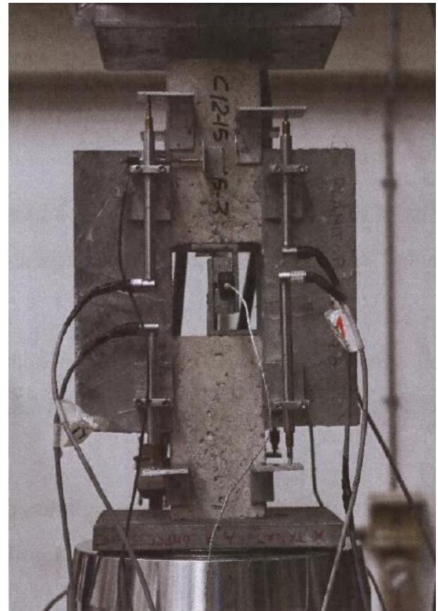
Figura 4. Ensayo de adherencia por rasante
