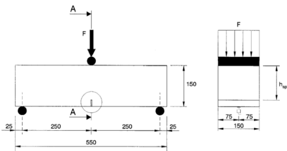
Figura 1. Ensayo de flexotracción según EN 14651
