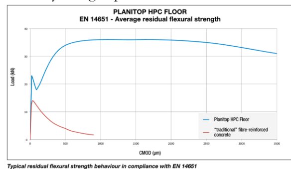
Figura 2. Diagrama del ensayo según EN 14651
