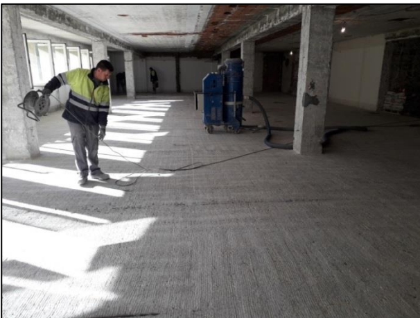
Figura 16. Estado final con la rugosidad requerida
