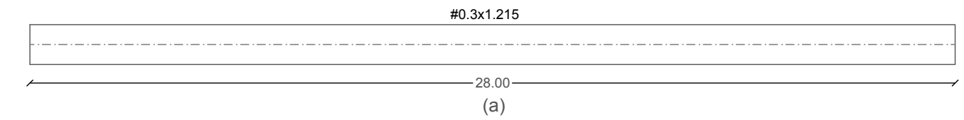
Figura 2. Detalles del diseño de (a) la cercha de hormigón reforzado, (b) la viga aligerada de hormigón pretensado y (c) la viga de hormigón pretensado.
