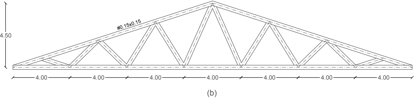
Figura 3. Detalles del diseño de (a) la viga de madera y (b) la cercha de madera.
